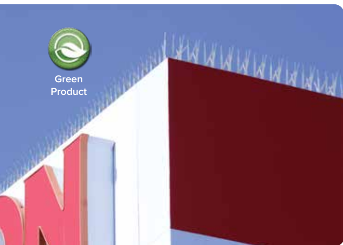
Los picos instalados a lo largo de las líneas del techo y cornisas evitarán que las aves se posen.
