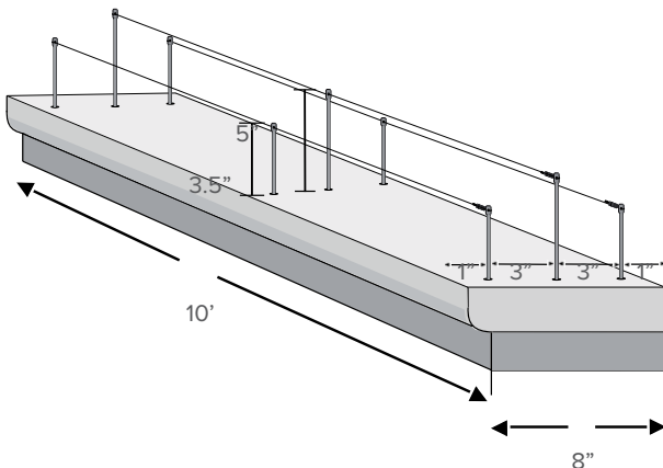
Bird Wire instalado en repisas de ventanas
